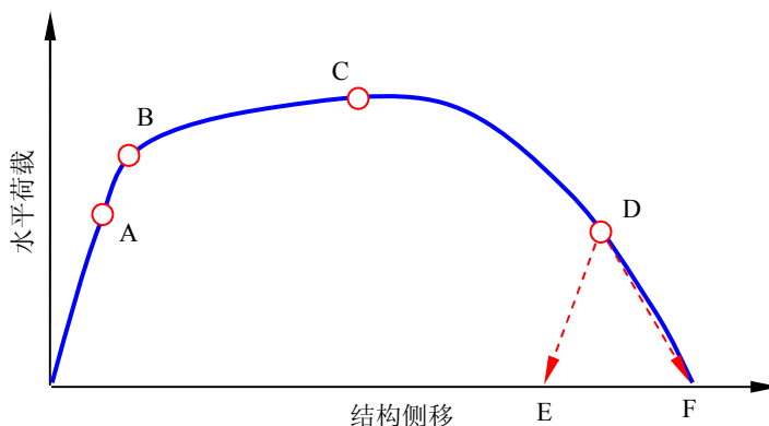
图 11 结构的抗侧行为
